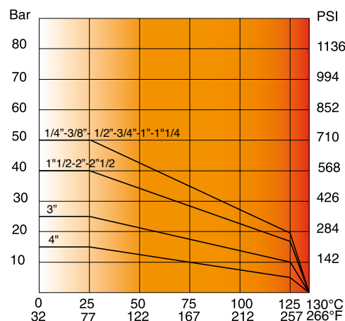
Diagramma pressione/temperatura
